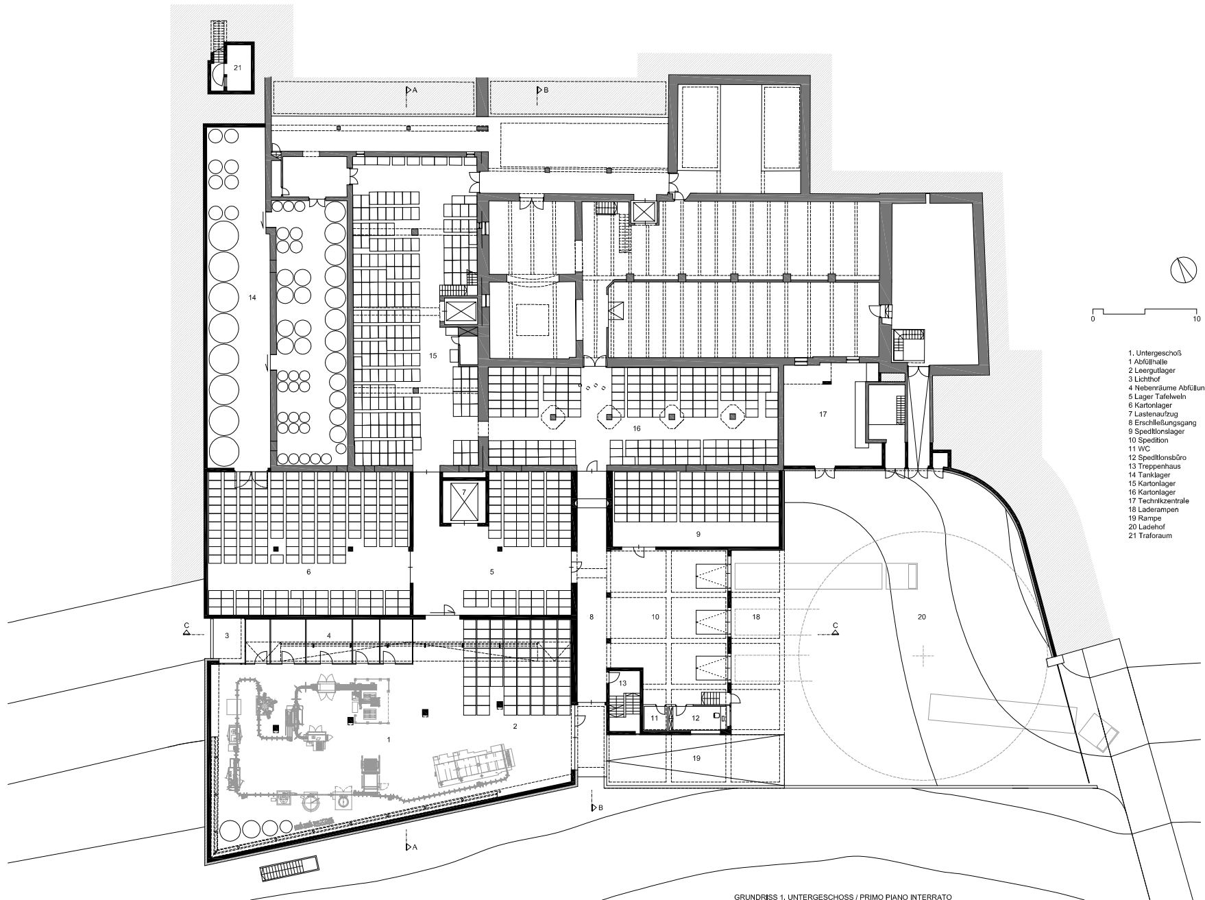
GRUNDRISS 1. UNTERGESCHOSS / PRIMO PIANO INTERRATO
